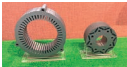
ステータコア(左)、ロータコア(右)
